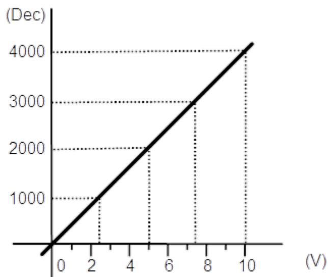
转换特性图:
