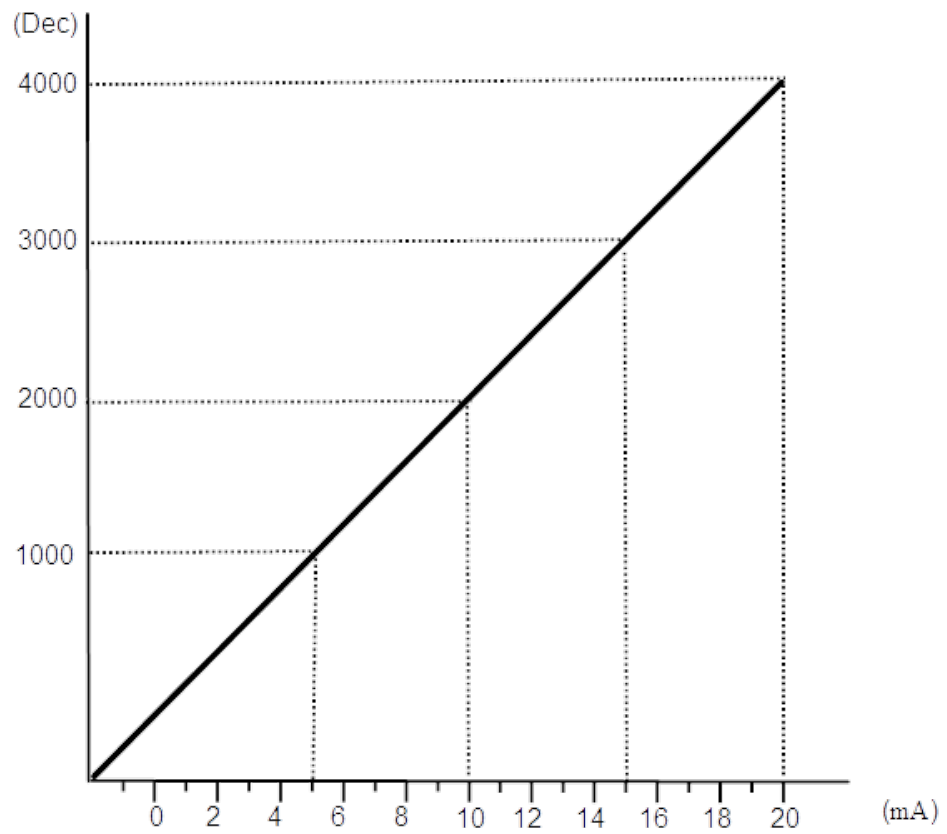
转换特性图:
